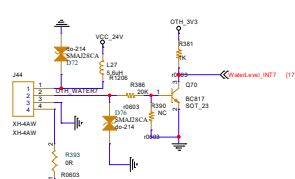
液位检测7
