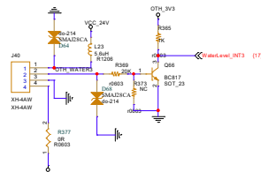
液位检测3
