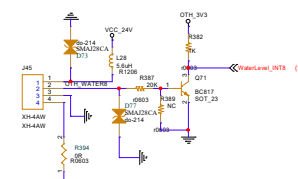
液位检测8
