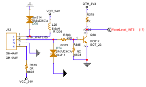
液位检测5
