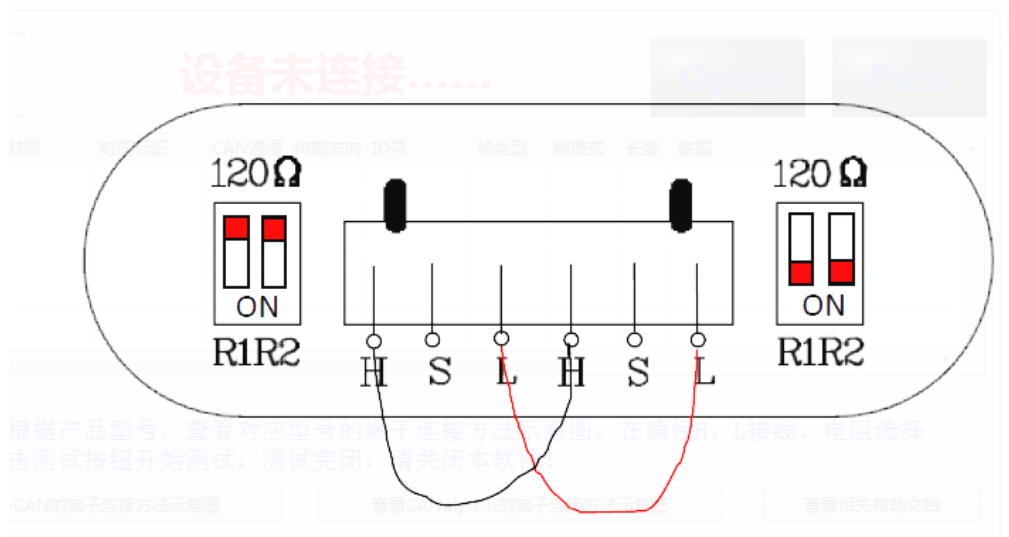
图 1 CANalsyt-II 分析仪测试接线图
