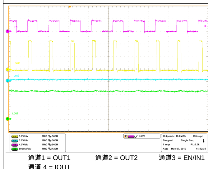
图 28. 带电流斩波的驱动器 PWM 运行
