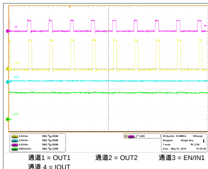
图 26. 驱动器 PWM 运行 (PH/EN)
